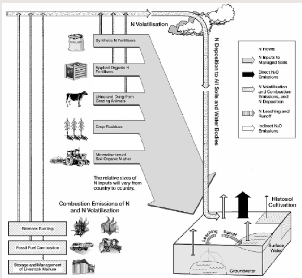
Figura 1 - Diagrama que ilustra as fontes e vias de N que resultam em emissões diretas e indiretas de N_2O pelo manejo de solos
