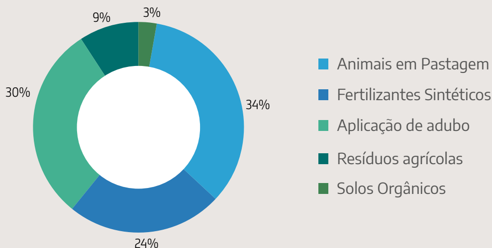
Figura 2 - Contribuição de cada categoria de emissão, em termos percentuais, do subsetor Solos Manejados (emissões diretas e indiretas).
