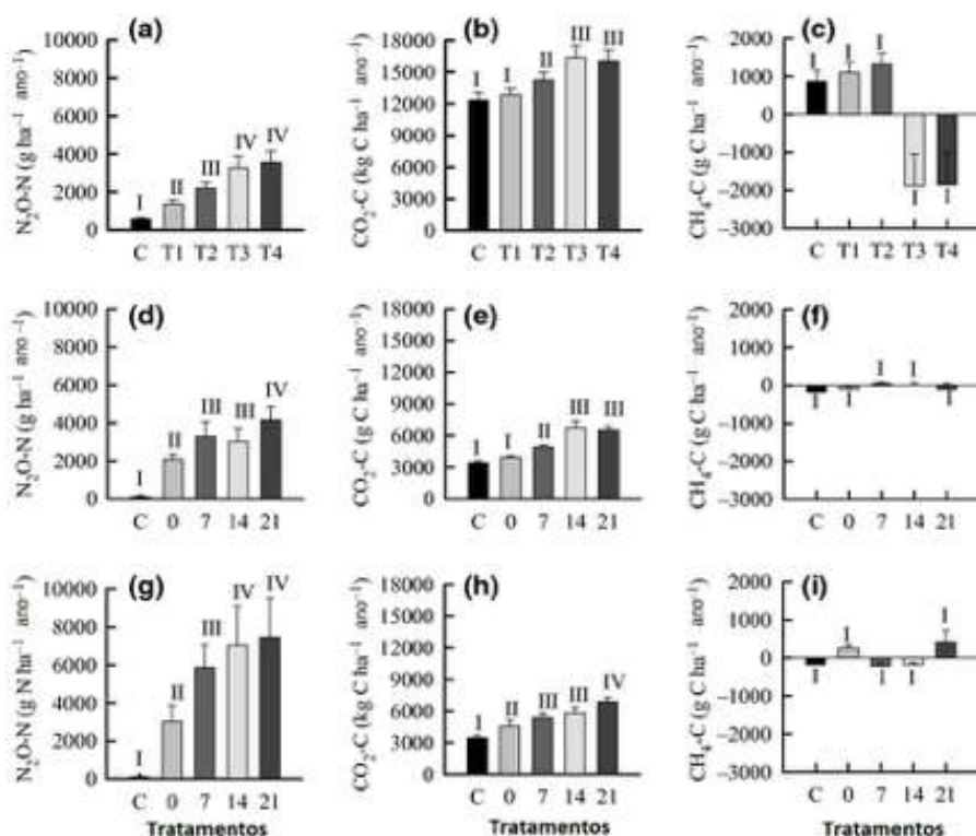
Figura: Fluxos cumulativos de N_2O , CO_2 e CH_4 em cana-planta (Jaú-SP) e cana-soca (Piracicaba-SP)
