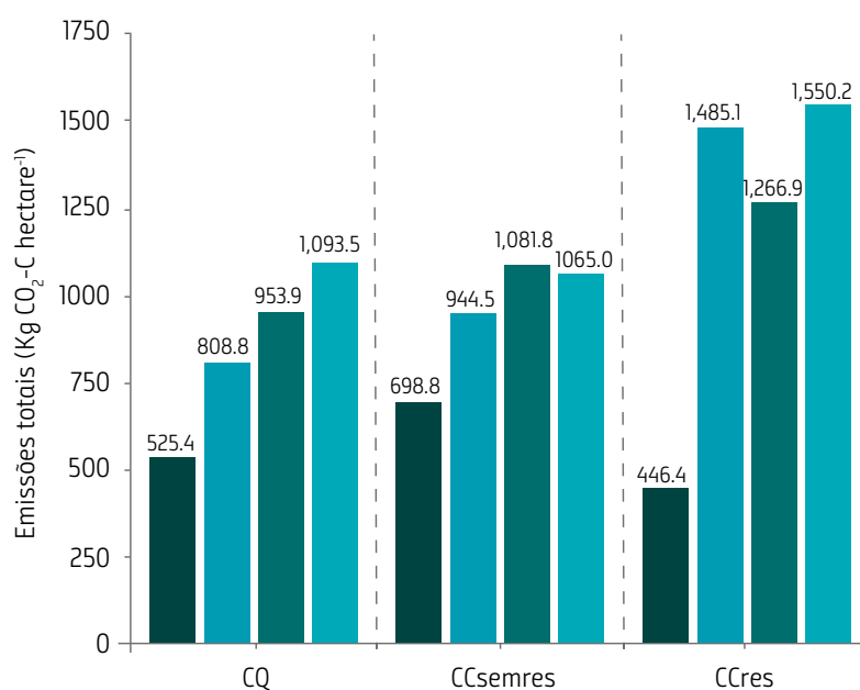
Figura 1: Emissões totais de carbono, considerando os sistemas de colheita da cana-de-açúcar queimada (CQ), colheita crua com resíduos removidos (CCsemres) e colheita crua com resíduos na superfície do solo (CCres) e seus respectivos manejos.
